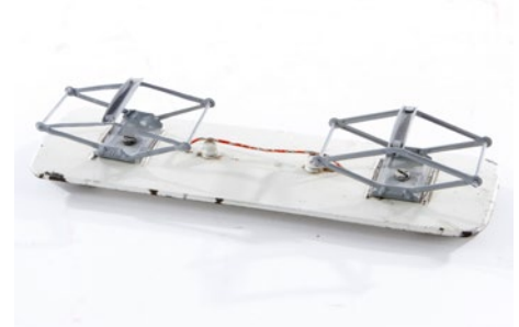
1240 Märklin Dach für E-Lok, Spur 0, Pantographen ersetzt, LS, L 17,5, als Ersatzteil 10,- €
