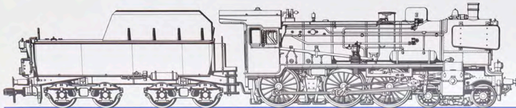
Personenzuglokomotive mit Wannentender
