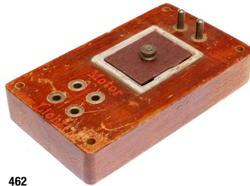
462 Märklin Sicherungskasten 5502/1342, uralt, Holzbock mit 2 Steckern und 4 Buchsen, dazwischen Porzellan-Sicherungskasten, Alterungsspuren, L 10, Z 2-3 50,- €
