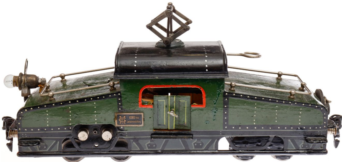
87 Märklin Vollbahnlok CL 3020, Spur 0, uralt, Starkstrom, grün, mit 1 el. bel. Stirnlampe, Pufferbohle und tw Rahmenbereiche nachlackiert, LS tw ausgebl., gealterter Lack, 1 Messingschild fehlt, sonst noch Z 2-3 1.800,- €
