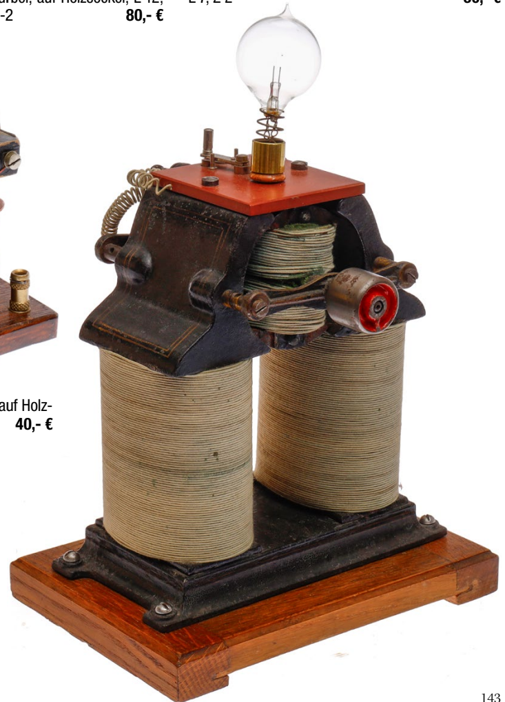
815 Kleiner Elektromotor, uralt, Holzausführung, auf Sockel, L 7, Z 2 30,- €
