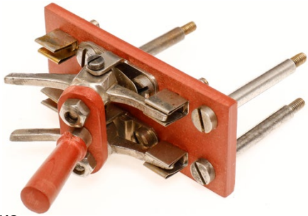
712 Märklin Replik Kippschalter für Starkstromlok, mit 3 Stiften, L 6 40,- €
